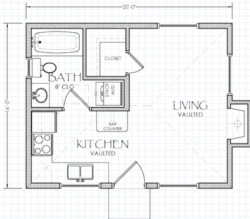
PLAN 320A 320 S.F.
